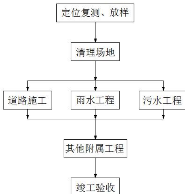
图 5-1 道路建设施工流程图
