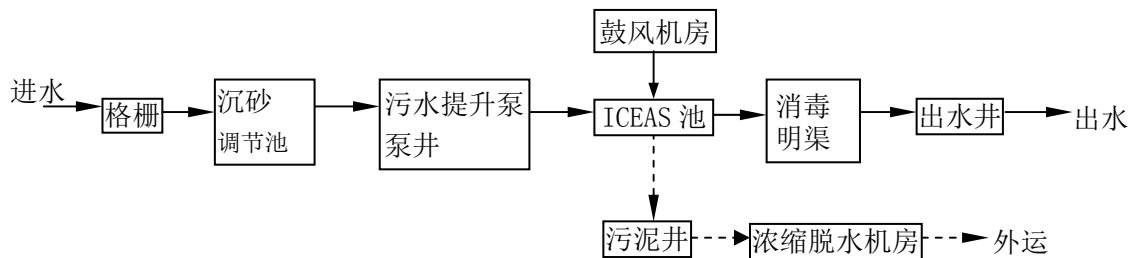
图 2 污水厂污水处理工艺流程图
